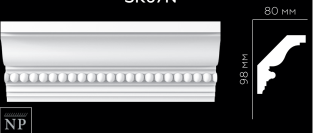
SK67N
